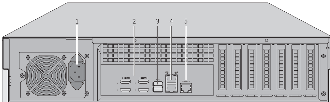
图1-3 TL-TUMS2600-N-SA后面板示意图
